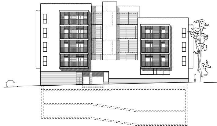
0 10 Façana nord Carrer Sant Gabriel
