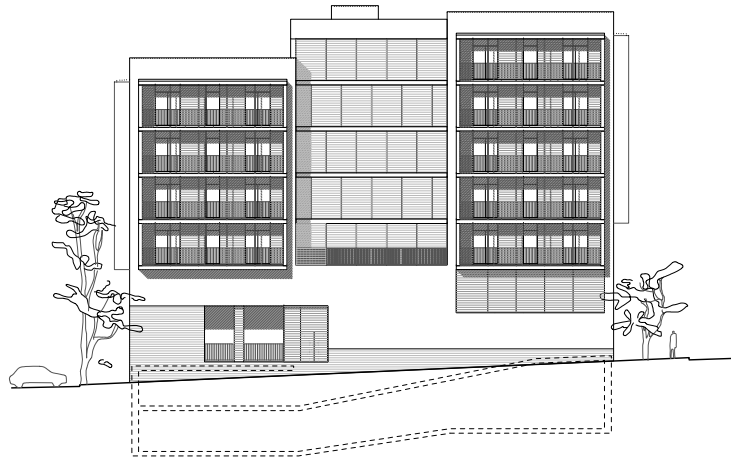
0 10 Façana sud Carrer Sant Jaume
