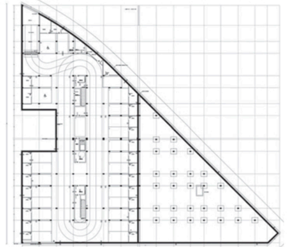
Planta de aparcamiento
