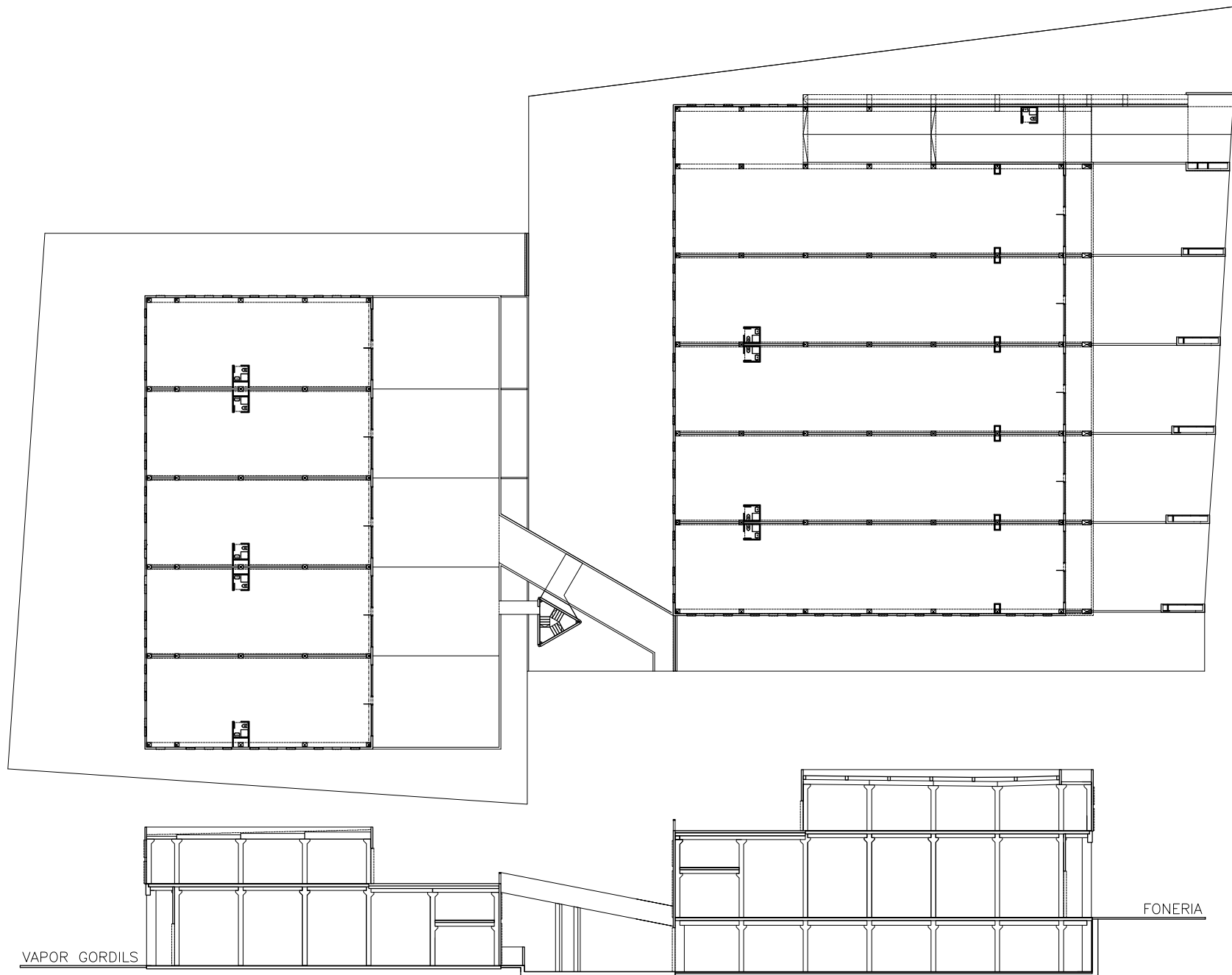
PLANTA BAIXA I PLANTA PRIMERA (FASE 1) PLANTA BAIXA CARRER FONERIA, 9 / PLANTA PRIMERA CARRER VAPOR GORDILS, 12 (FASE 2)
