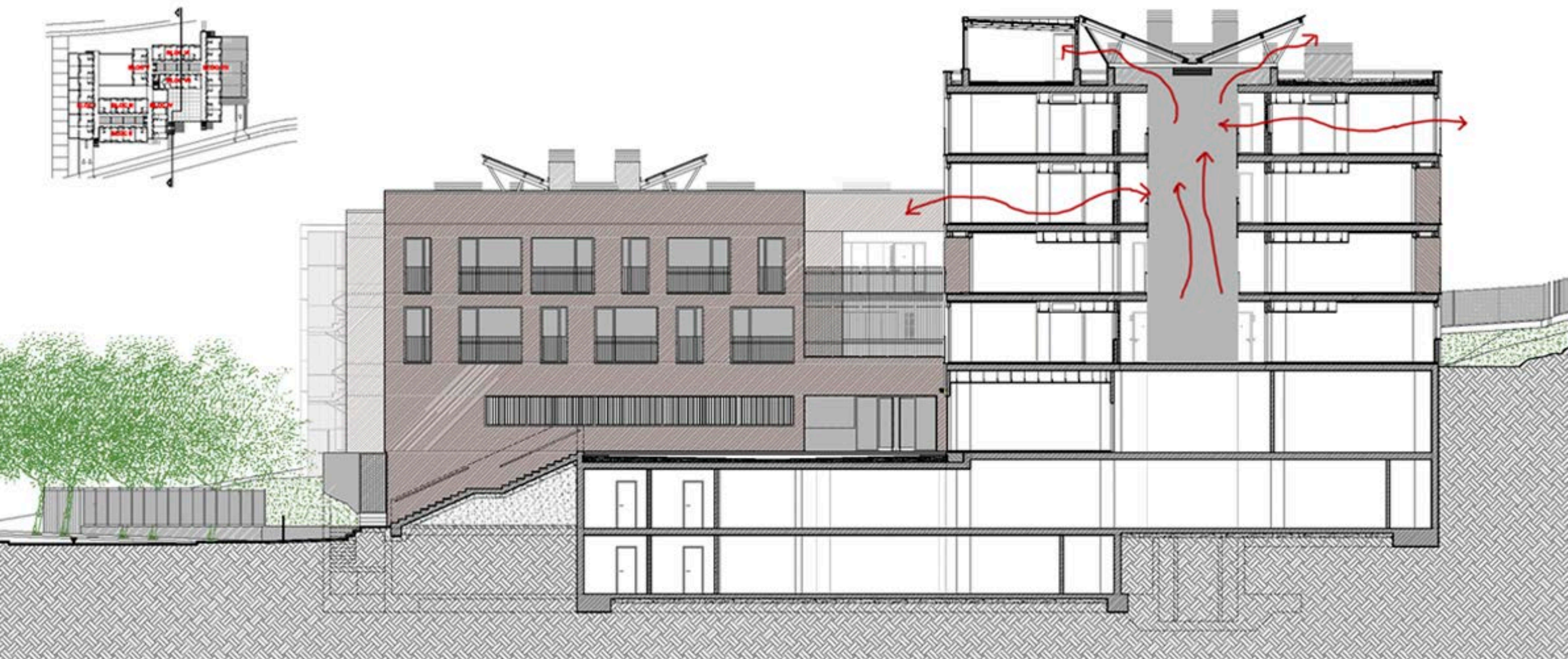
secció transversal
