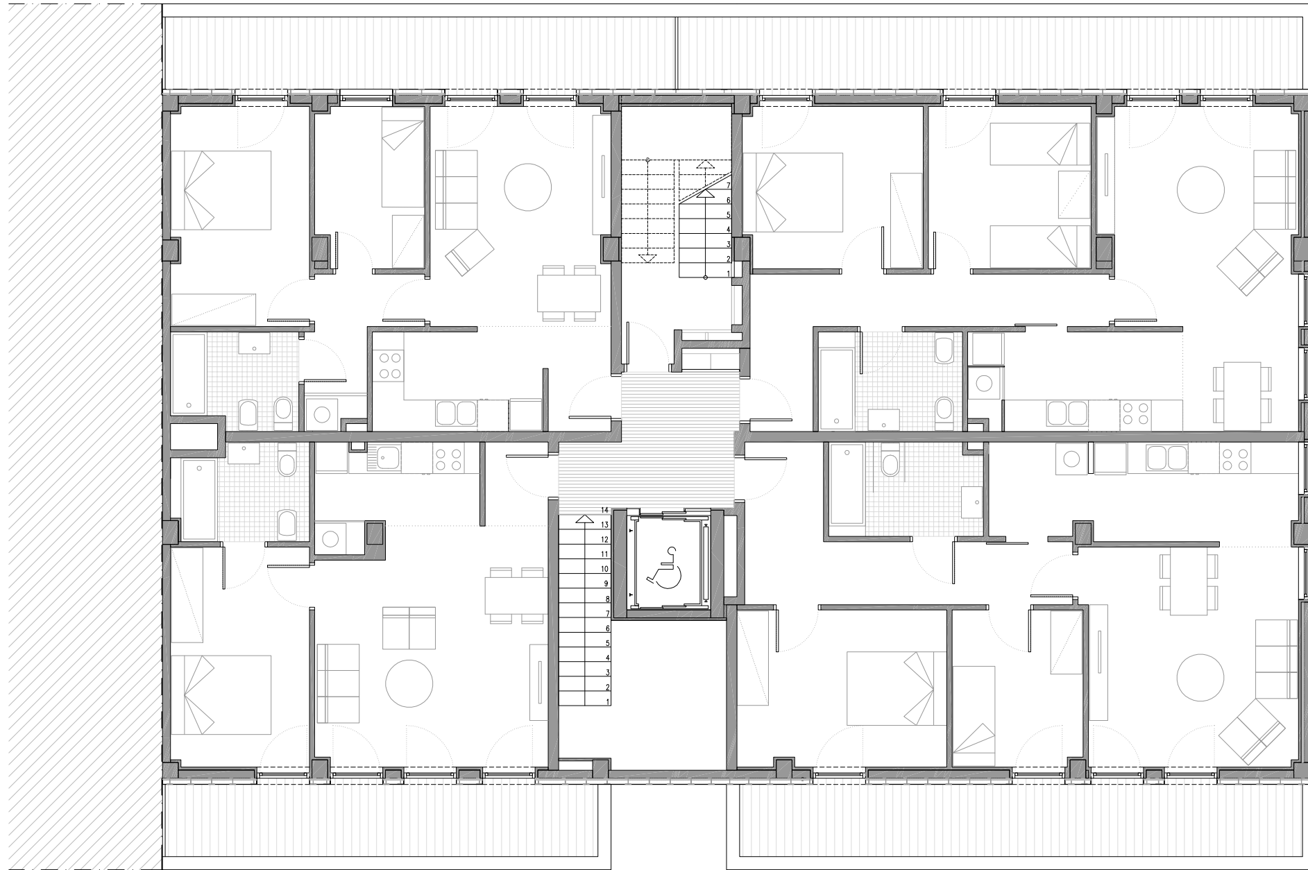
PLANTA BAIXA
