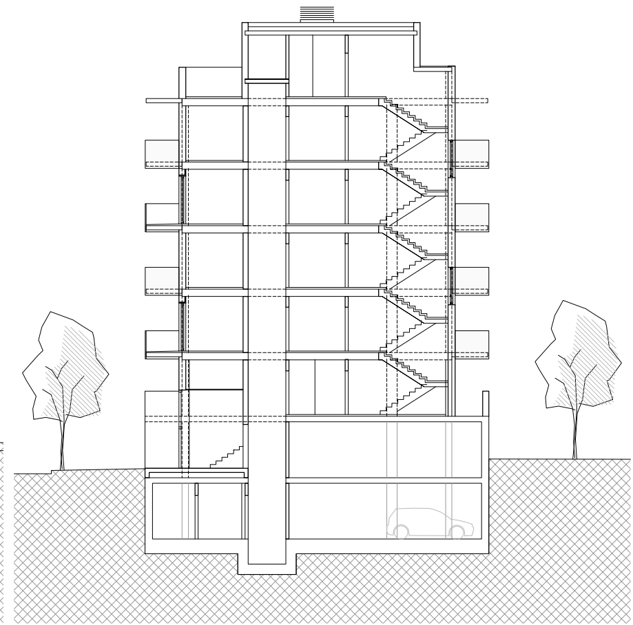
SECCIÓ TRANSVERSAL
