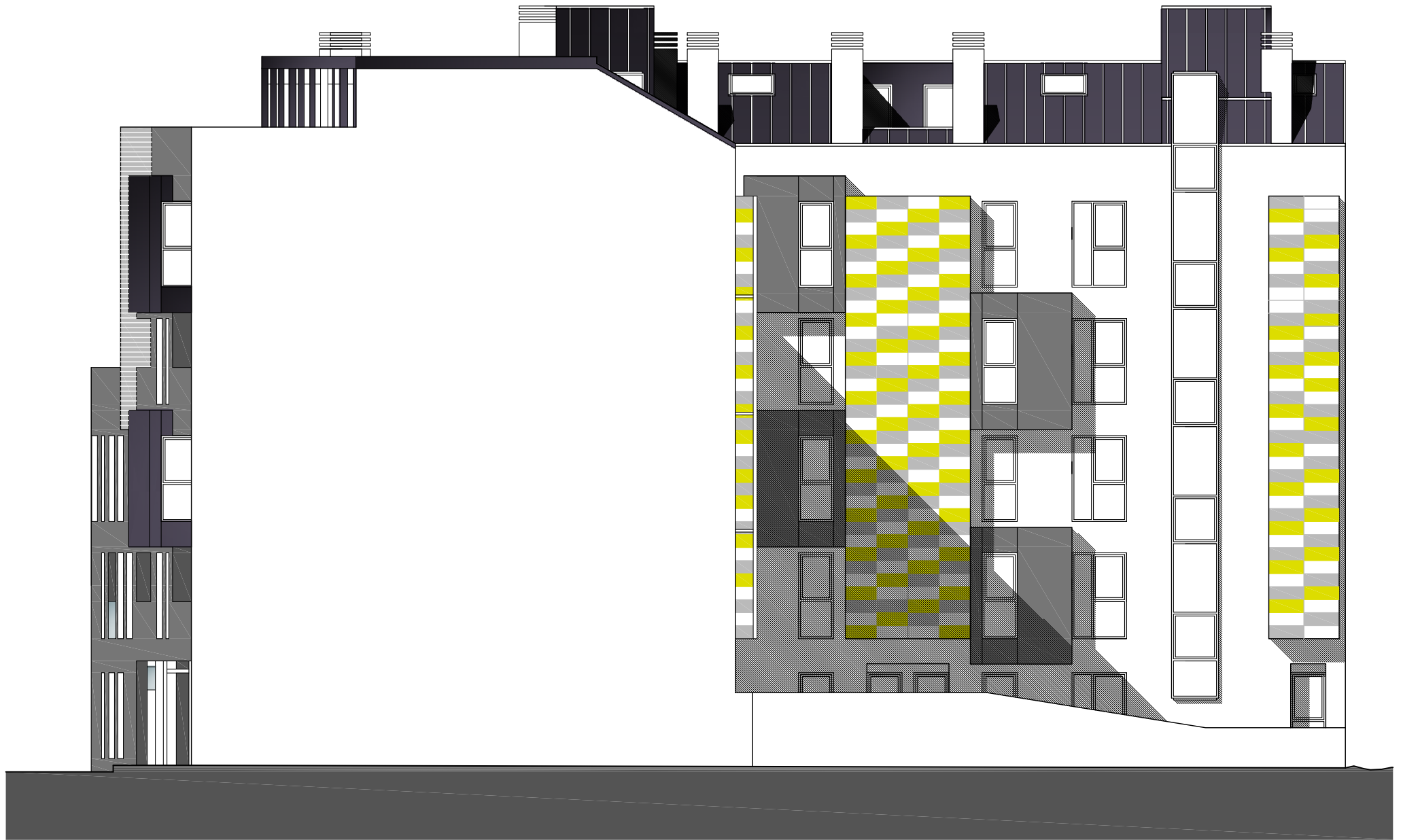
ALZADO SUR . Escala 1/125
