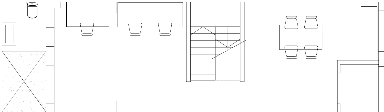
PLANTA BAIXA
