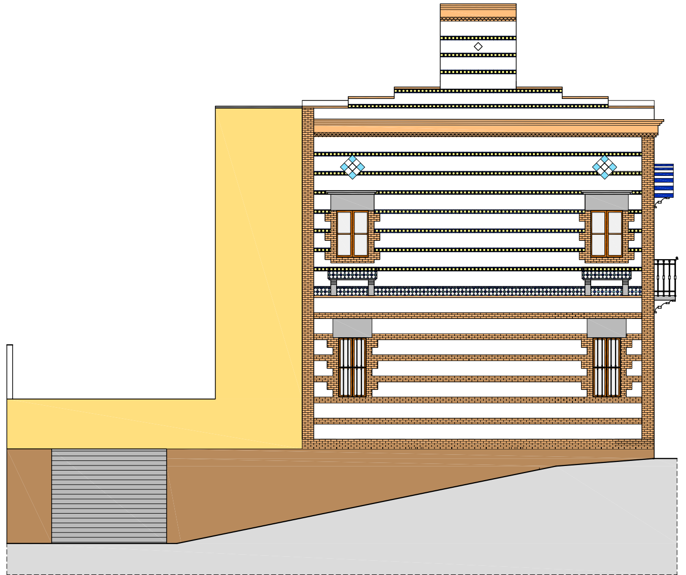
ALÇAT LATERAL
