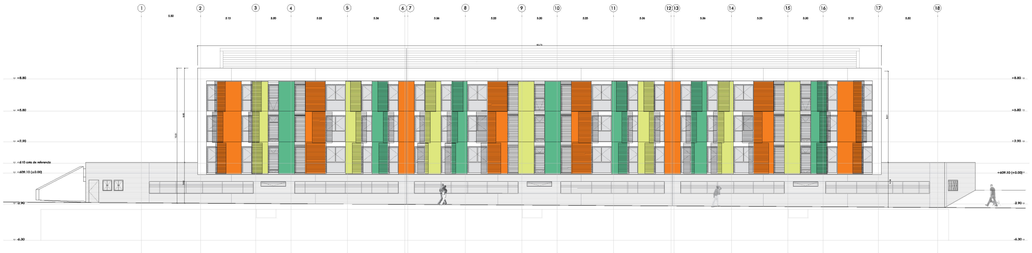
ALZADO SUR
