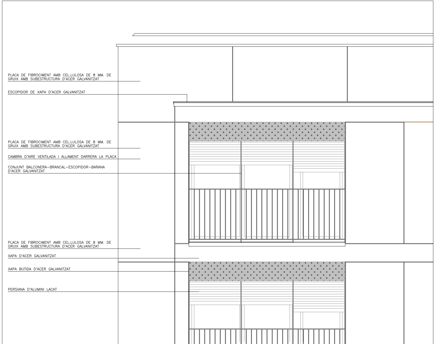
DETALLES FACHADA
