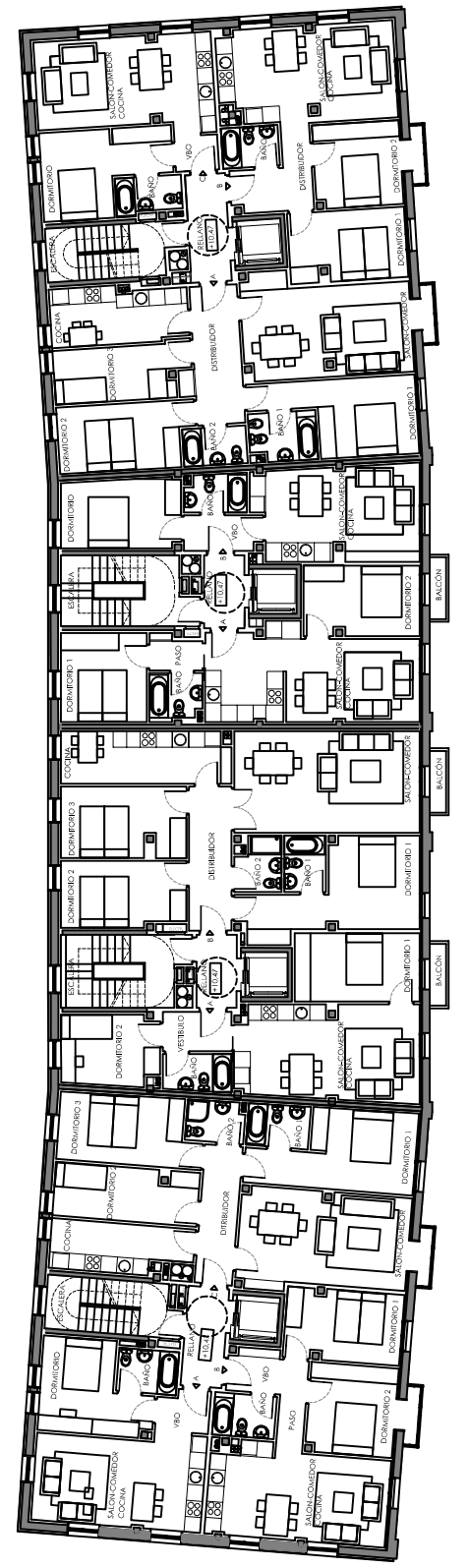
PLANTA TERCERA
