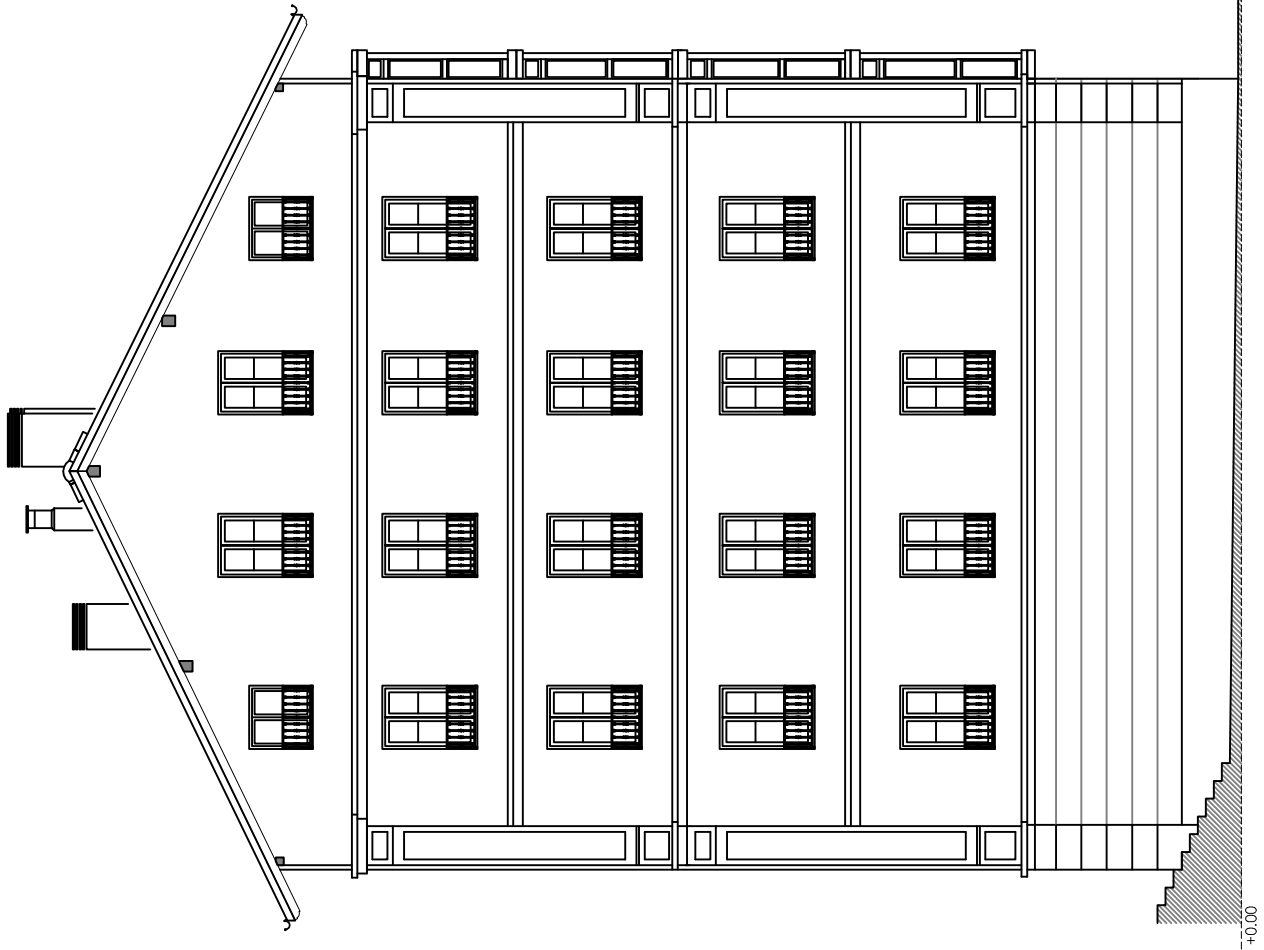
ALZADO ESTE
