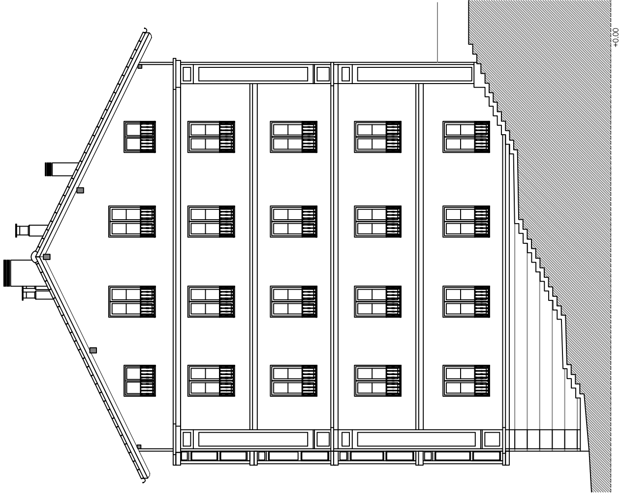
ALZADO OESTE
