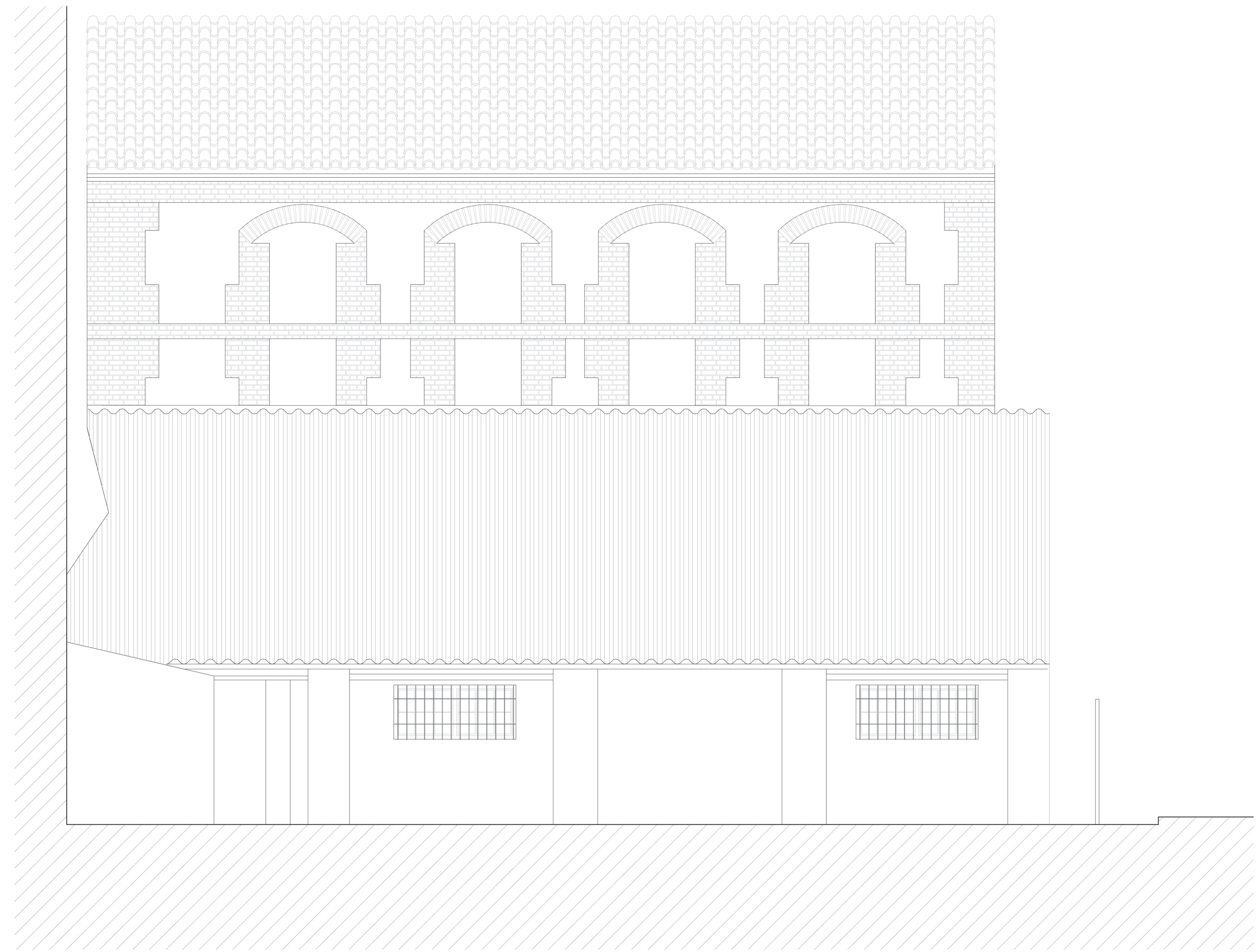
ALZADO EXTERIOR *A*
