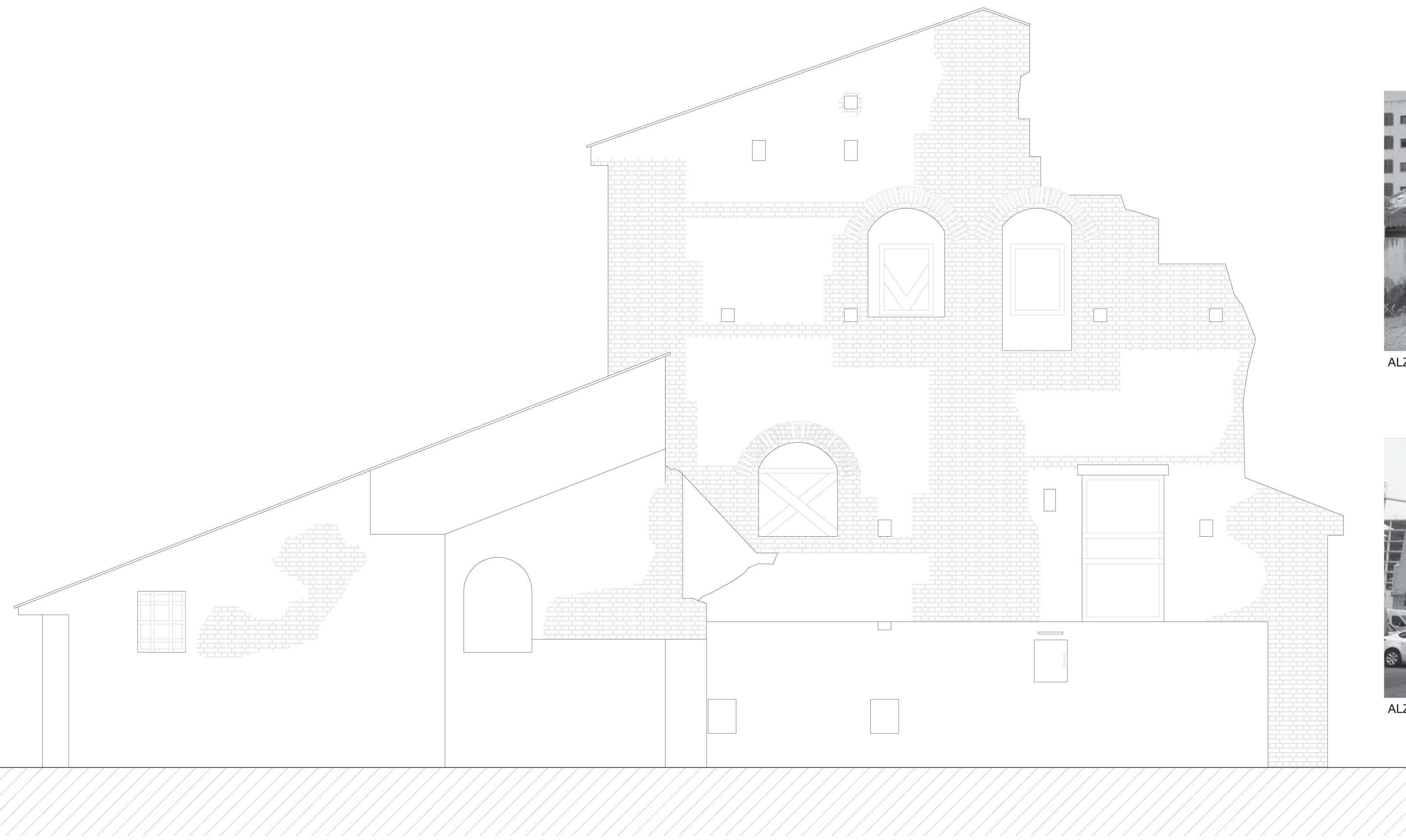
ALZADO EXTERIOR *B*
