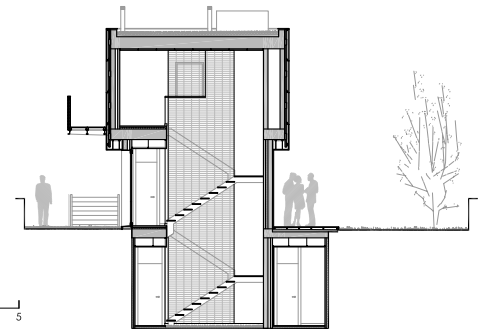
SECCIÓ F
