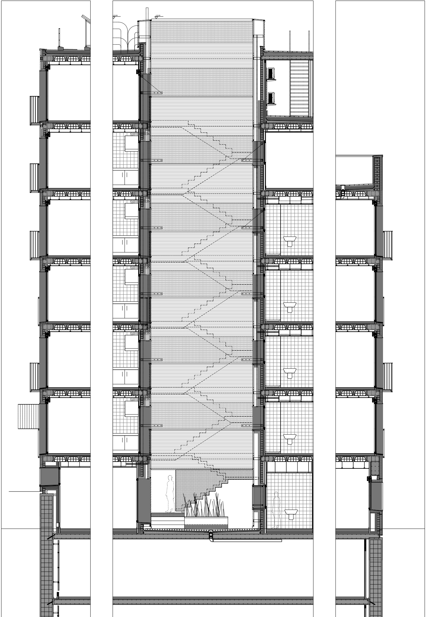
SECCION TRANSVERSAL POR HUECOS
