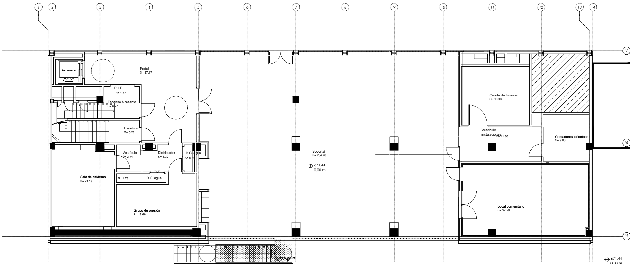
Planta Baja_Usos y superficies E: 1:100
