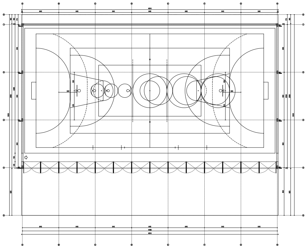
PLANTA A NIVELL DE PISTA
