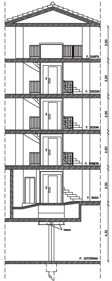
ALÇAT FRONTAL
