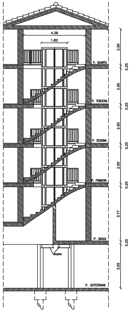
ALÇAT POSTERIOR
