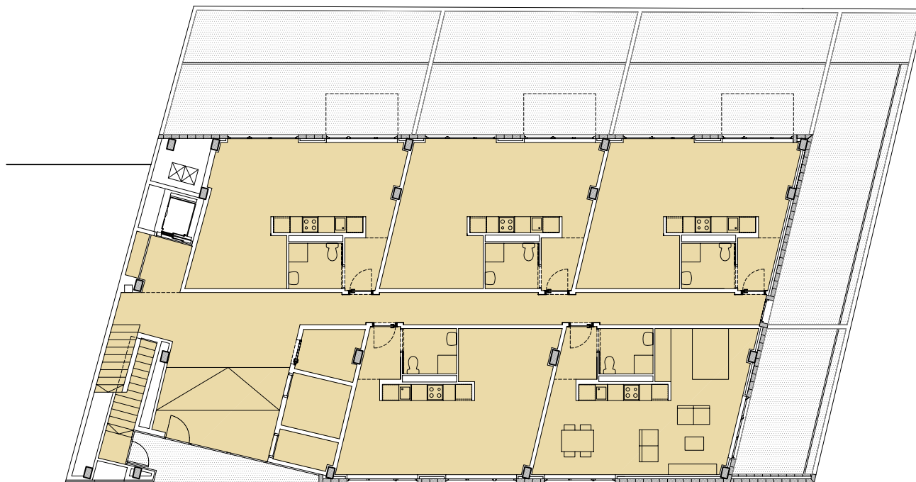
Planta baixa
