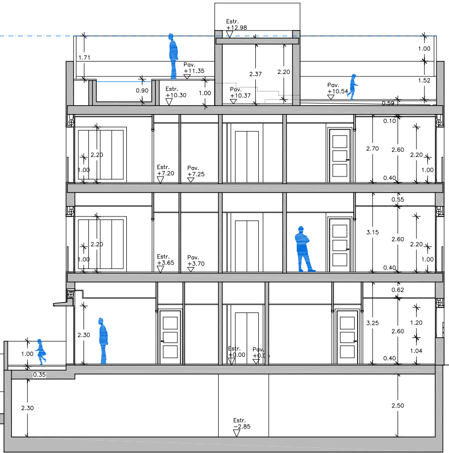
0 1 5 E: 1/150 SECCIÓ A-A'
