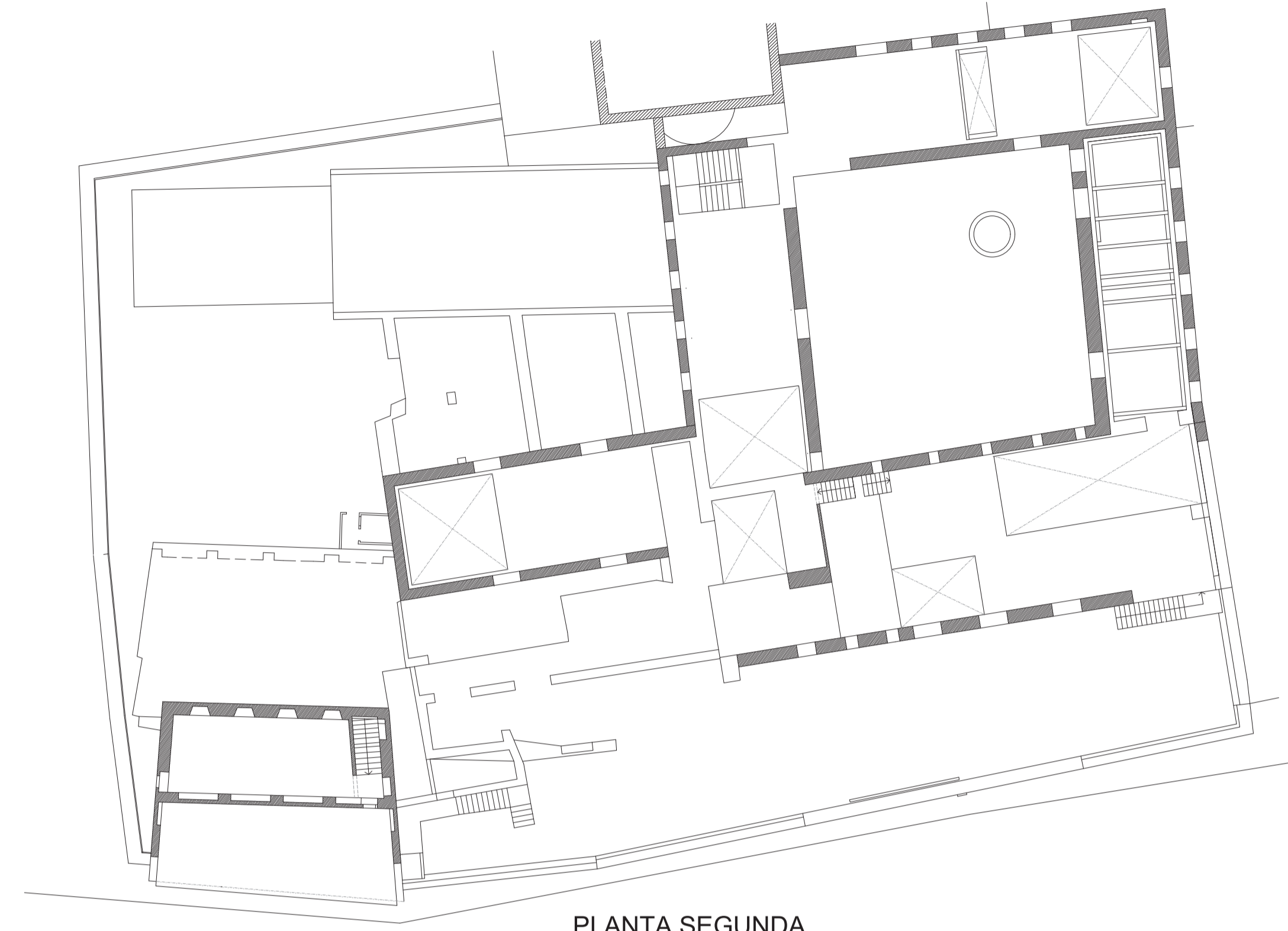
PLANTA SEGUNDA
