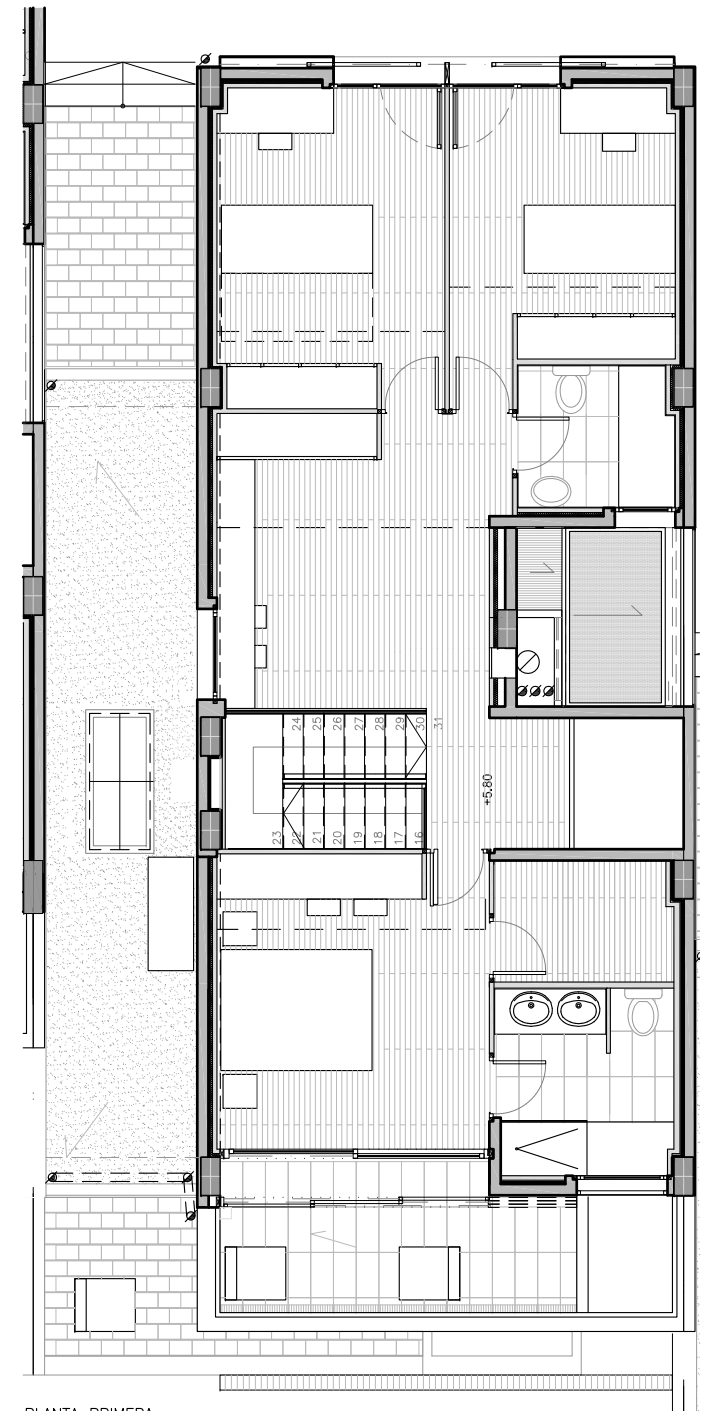
PLANTA PRIMERA S útil= 75.48m2
