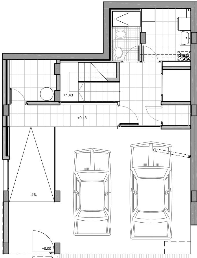
PLANTA SOTERRANI S útil= 72.04 m2
