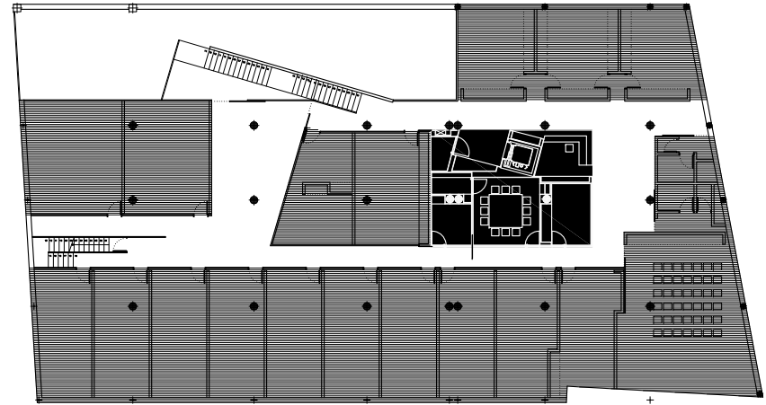
PLANTA. PROJECTE
