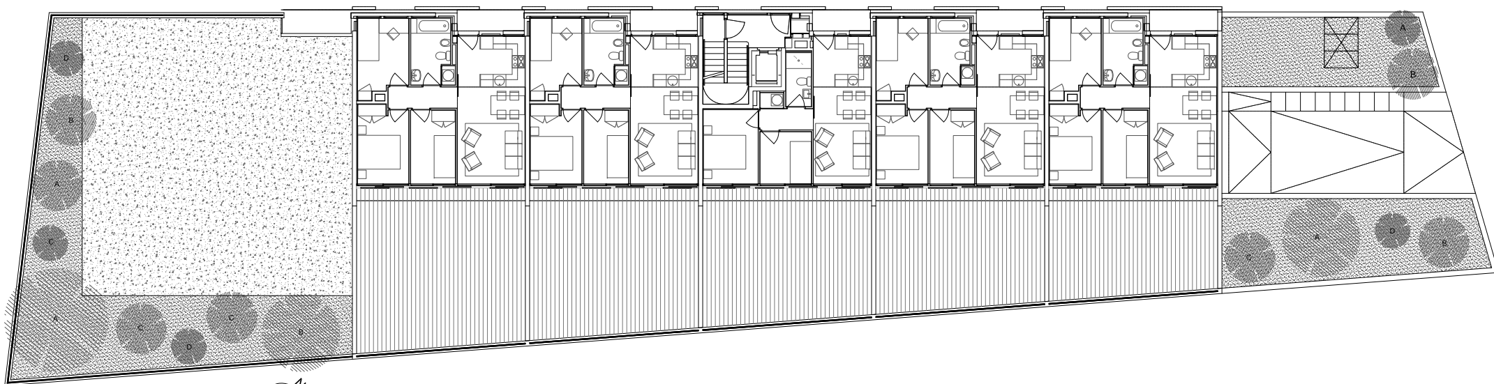
PLANTA BAIXA
