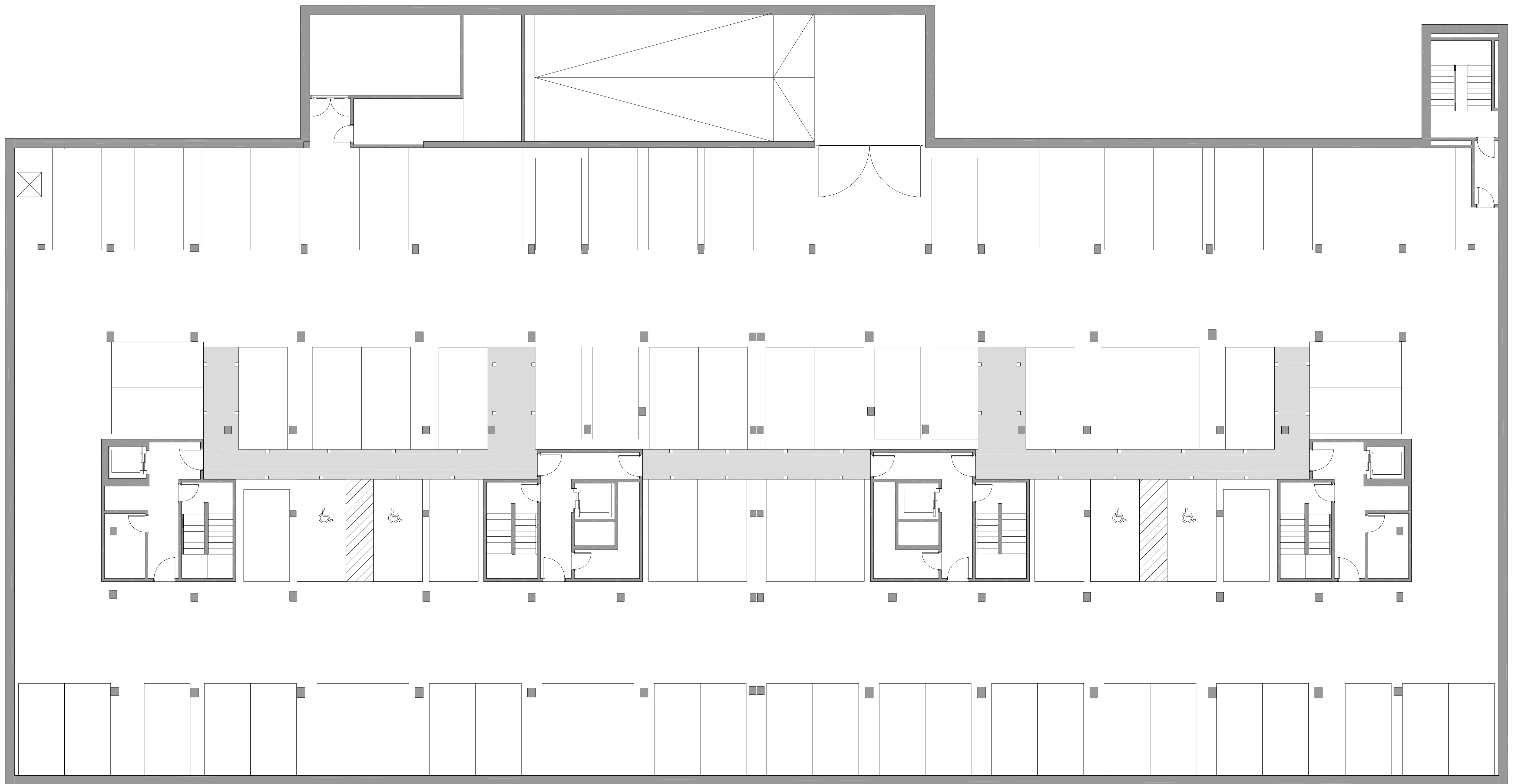
PLANTA SÓTANO -2
