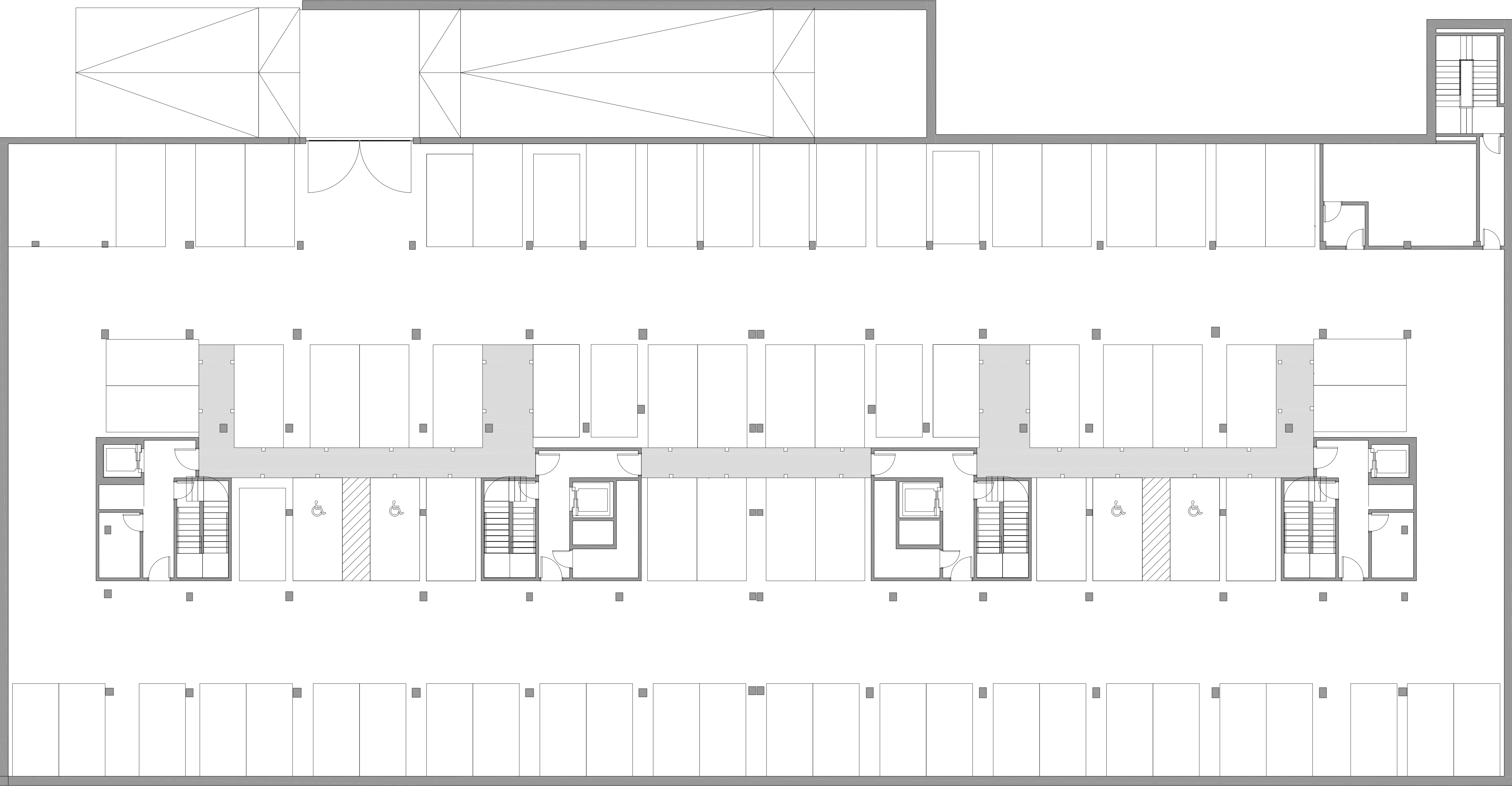
PLANTA SÓTANO -1
