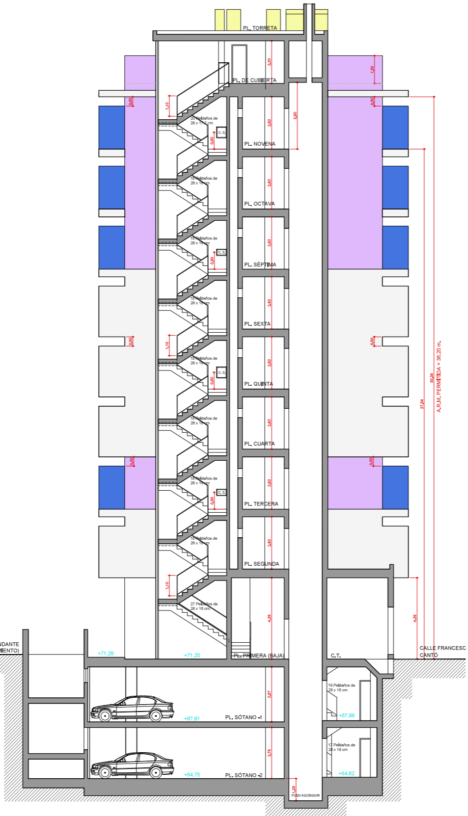
SECCIÓN C-D
