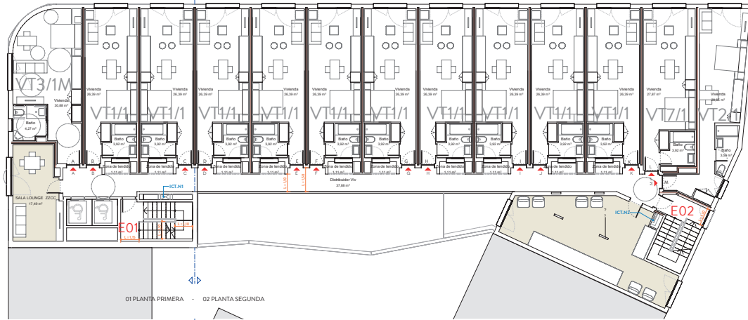
Planta Primera/Segunda
