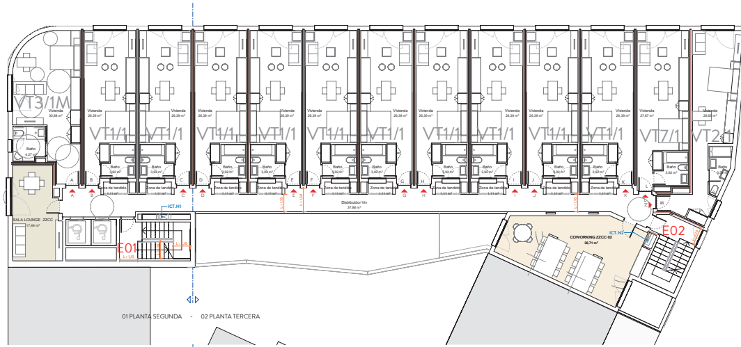
Planta Segunda/Tercera
