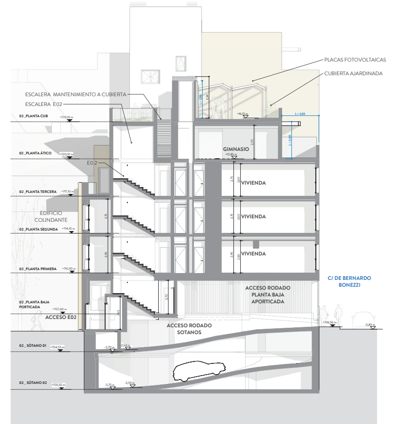
SECCIÓN 3 ACCESO RODADO
