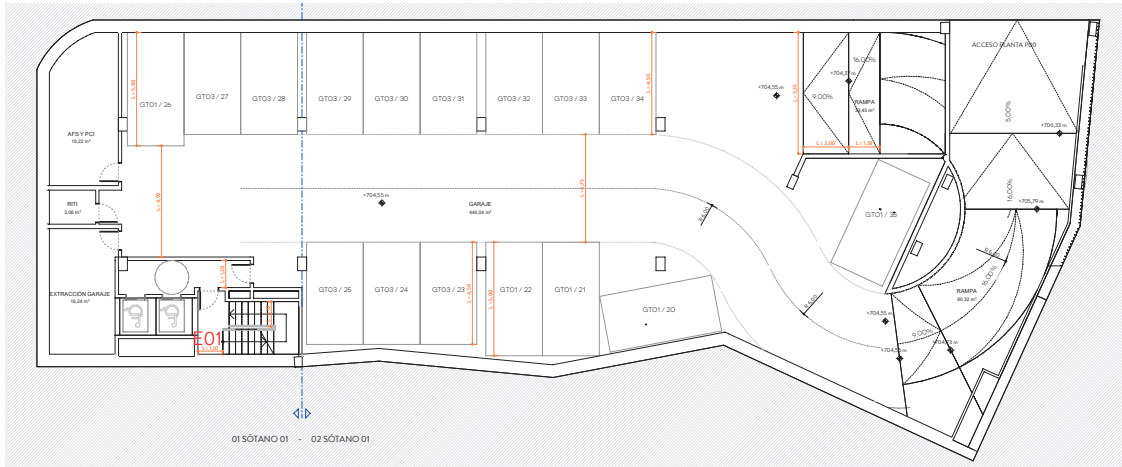
Planta Sótano 01
