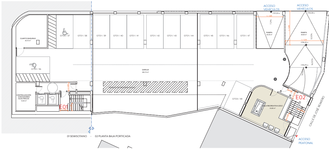
Semisótano/Planta Baja
