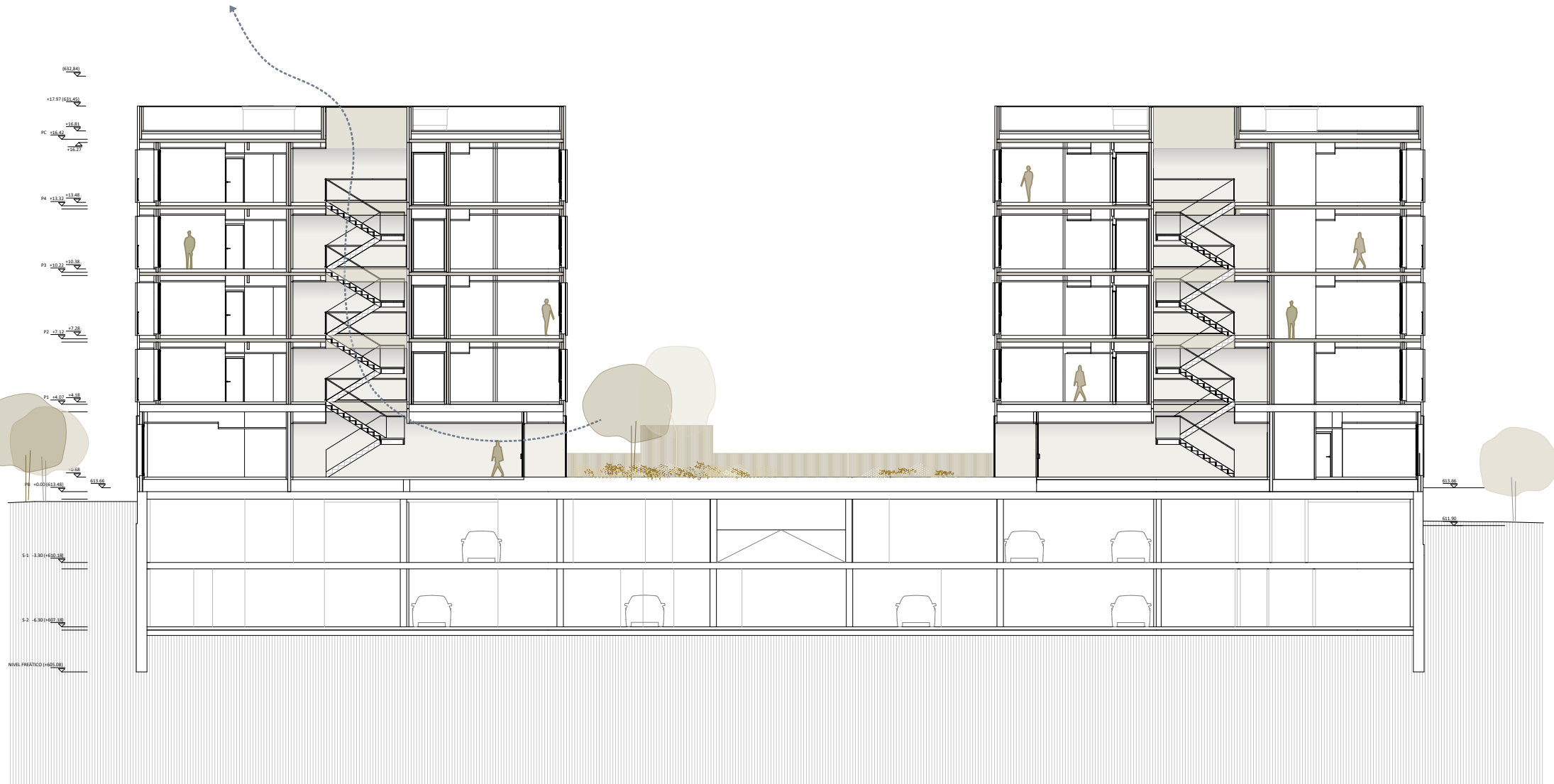
SECCIÓN LONGITUDINAL E: 1/250
