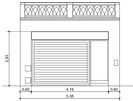
FAÇANA PARCEL-LA B "PASSEIG DELS ANGLESSOS 17"
