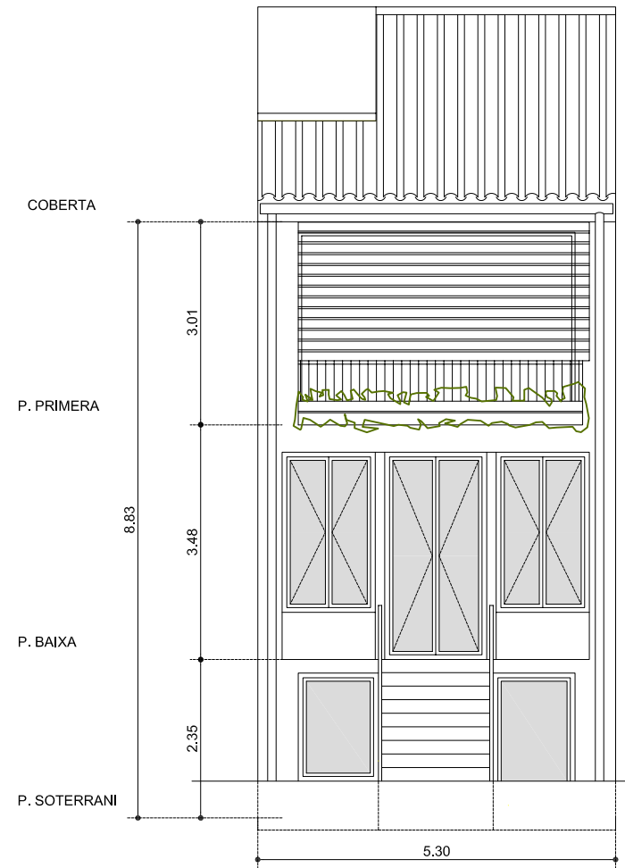
FAÇANA PARCEL-LA A "INTERIOR PATI"
