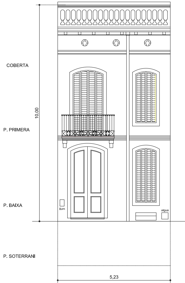
FAÇANA PARCEL-LA A "C/ CIUTAT DE LA PAZ 32"
