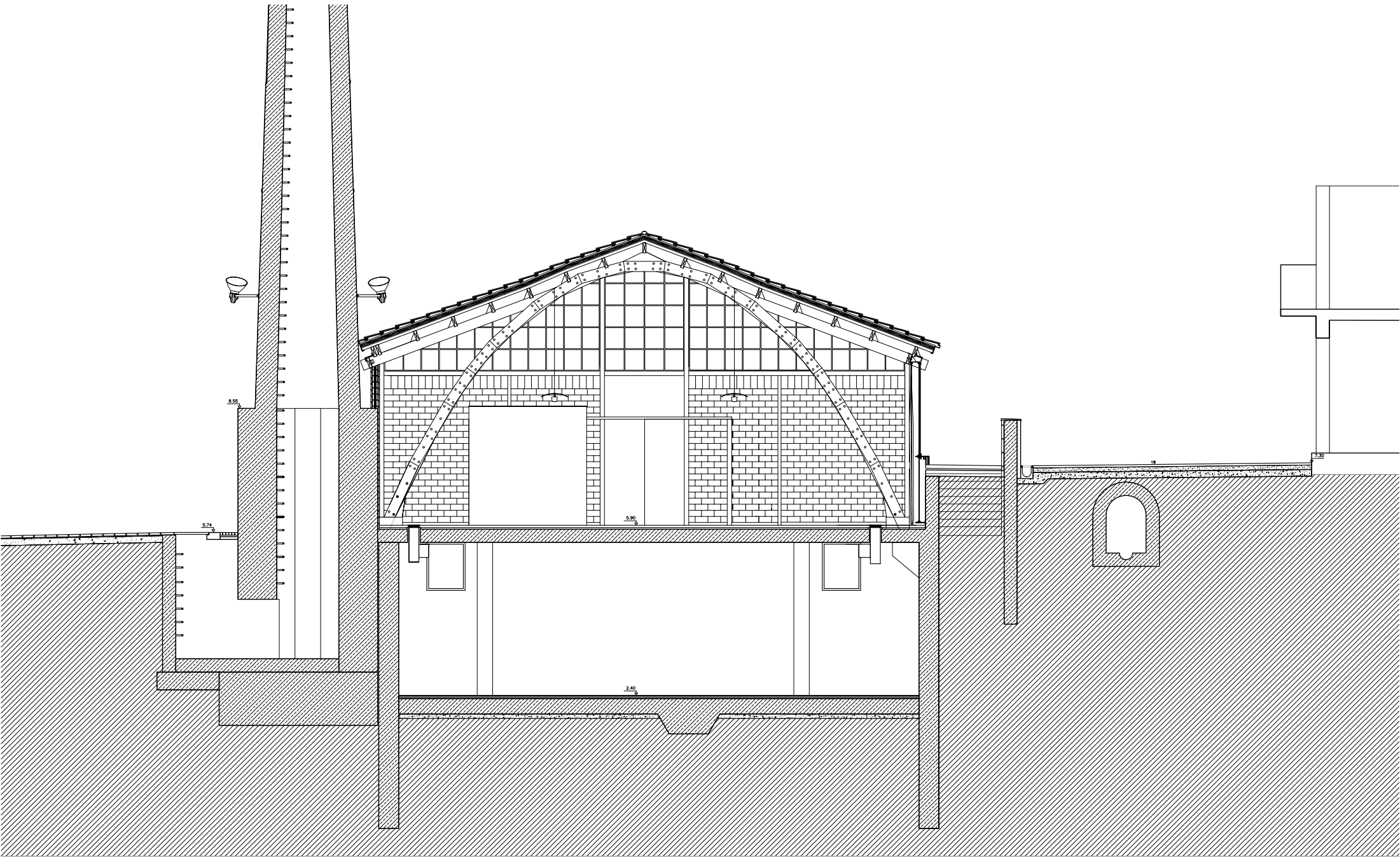
SECCIÓN TRANSVERSAL CON EL NUEVO SÓTANO PARA LOS NUEVOS SERVICIOS DE LA NAVE
