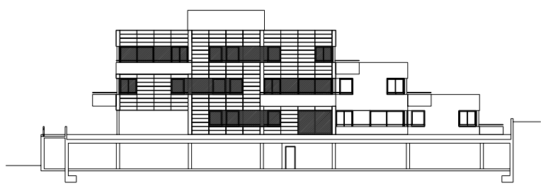
SECCIÓ TRANSVERSAL PER APARCAMENT 0 2 4 6 8 10m
