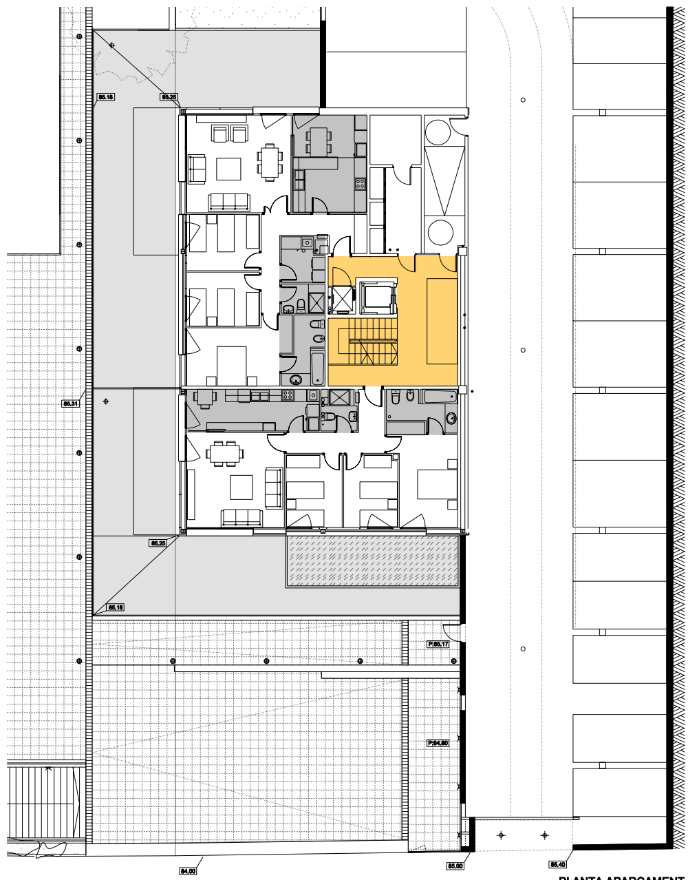
PLANTA APARCAMENT
