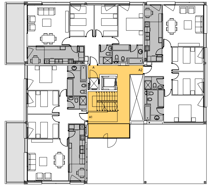
PLANTA BAIXA 0 1 2 3 4 5m N
