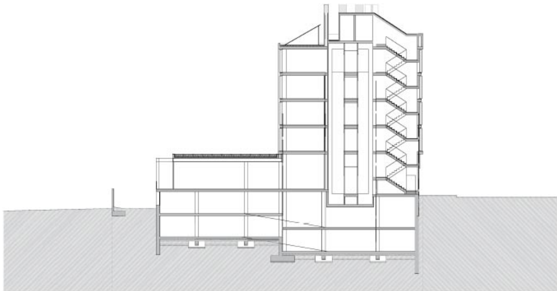
SECCIÓ LONGITUDINAL
