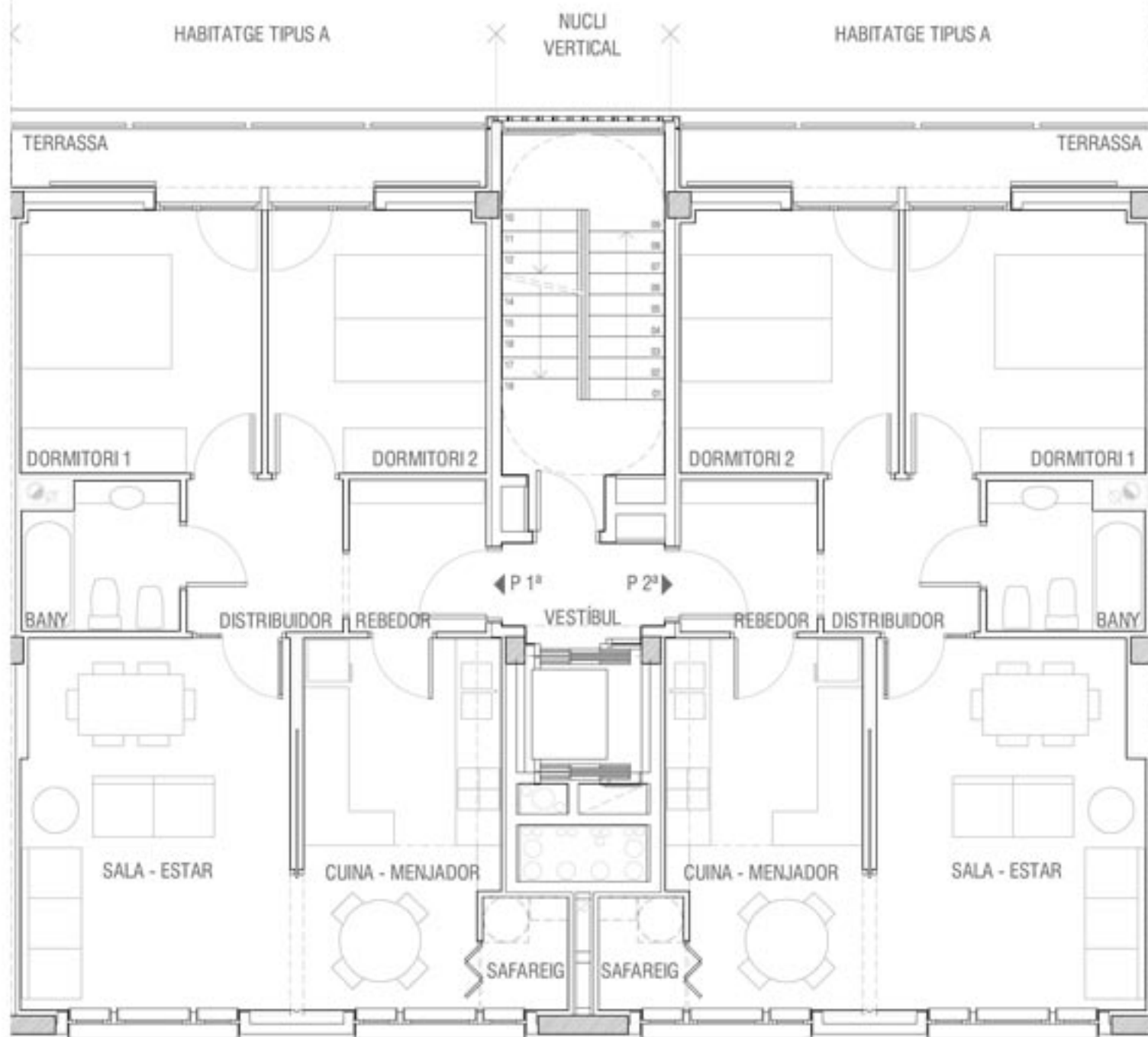
PLANTA D'HABITATGES TIPOLOGIA D'HABITAGES TIPUS A
