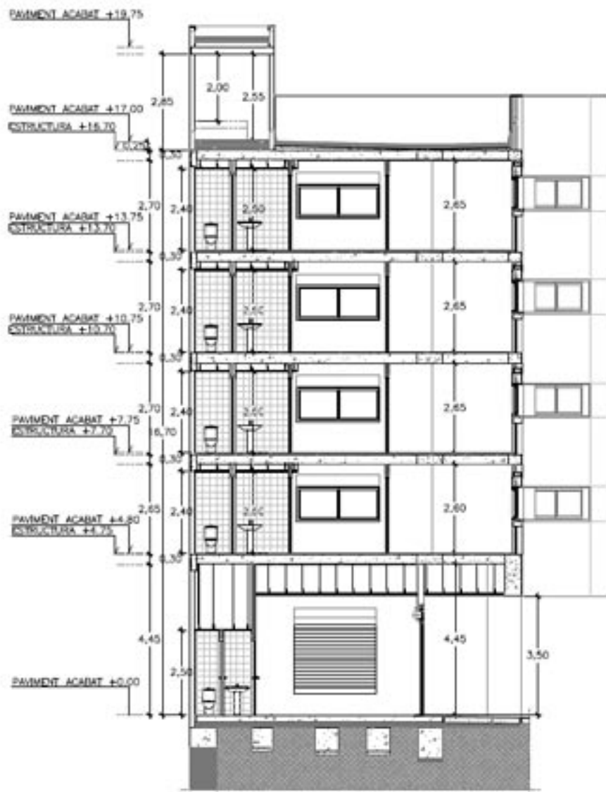
SECCIÓ B-B'
