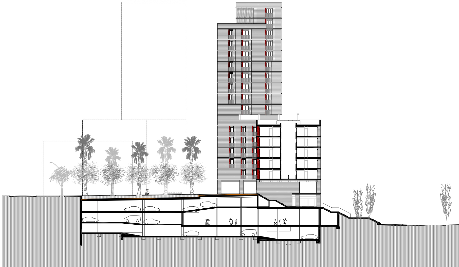
0 2.5 5 10m SECCIÓ TRANSVERSAL
