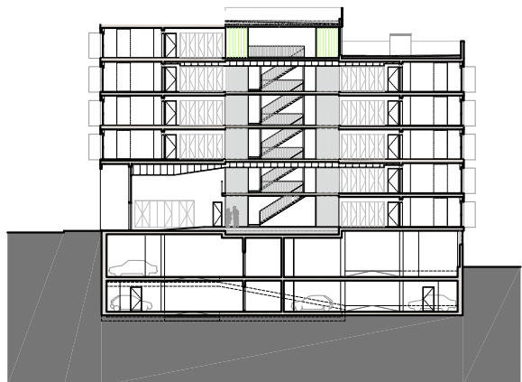
E 1/600 Dina4
