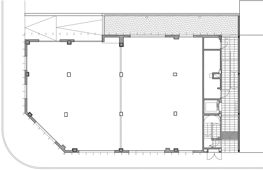
PLANTA BAIXA
