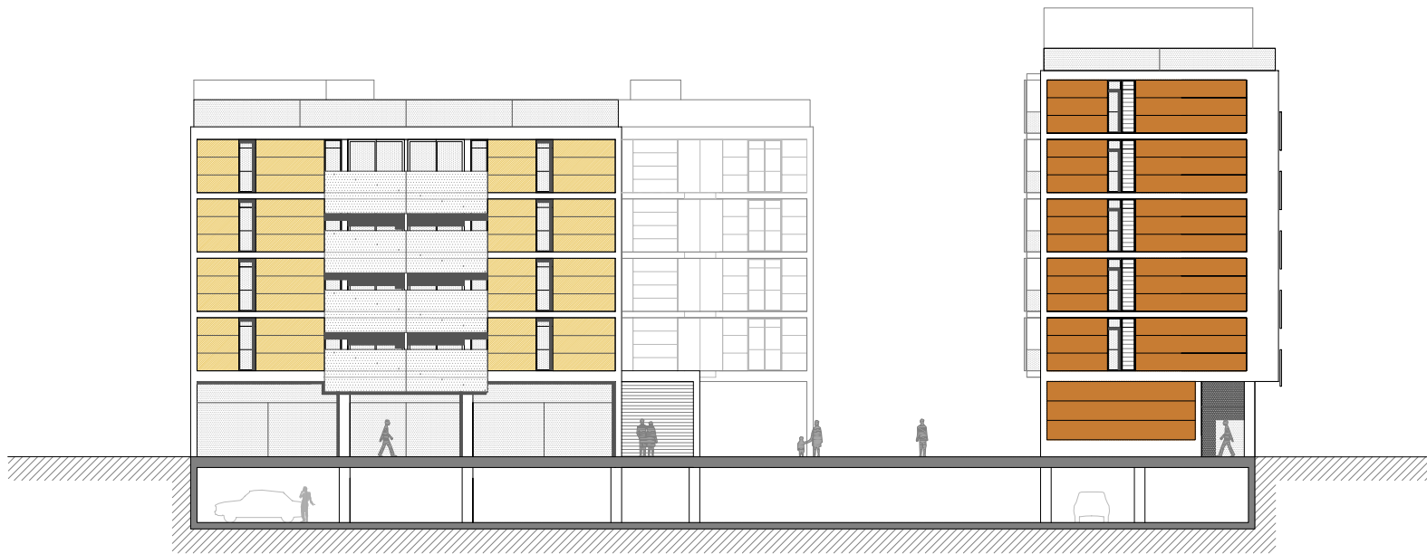
FAÇANA C/ MART
