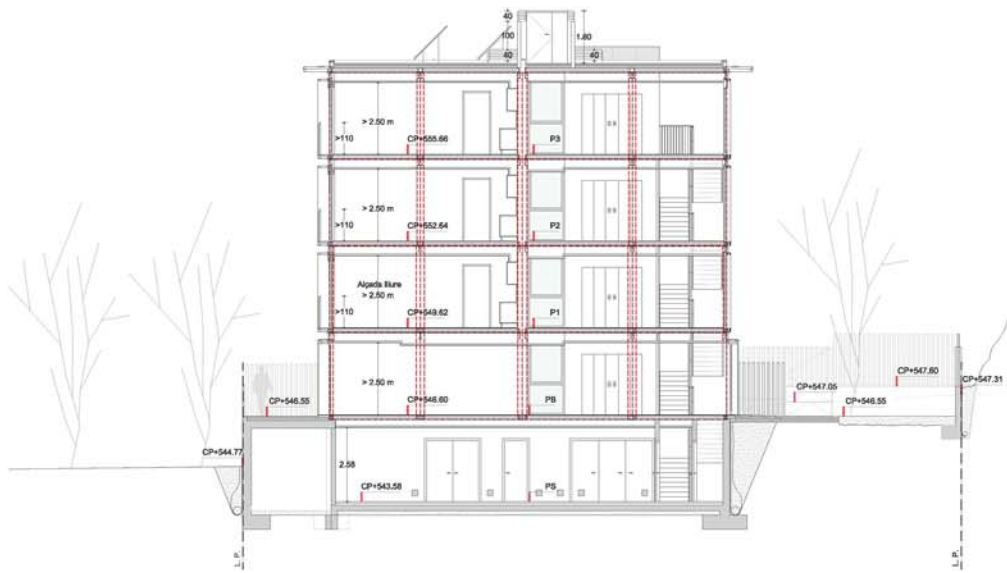
S2 SECCIÓ TRANSVERSAL E: 1/100
