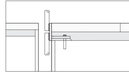
DETALLE FIJACIÓN BARANDILLA
