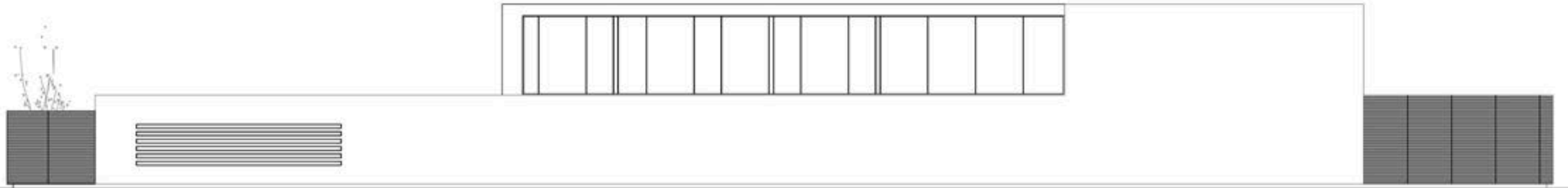
ALZADO ESTE
