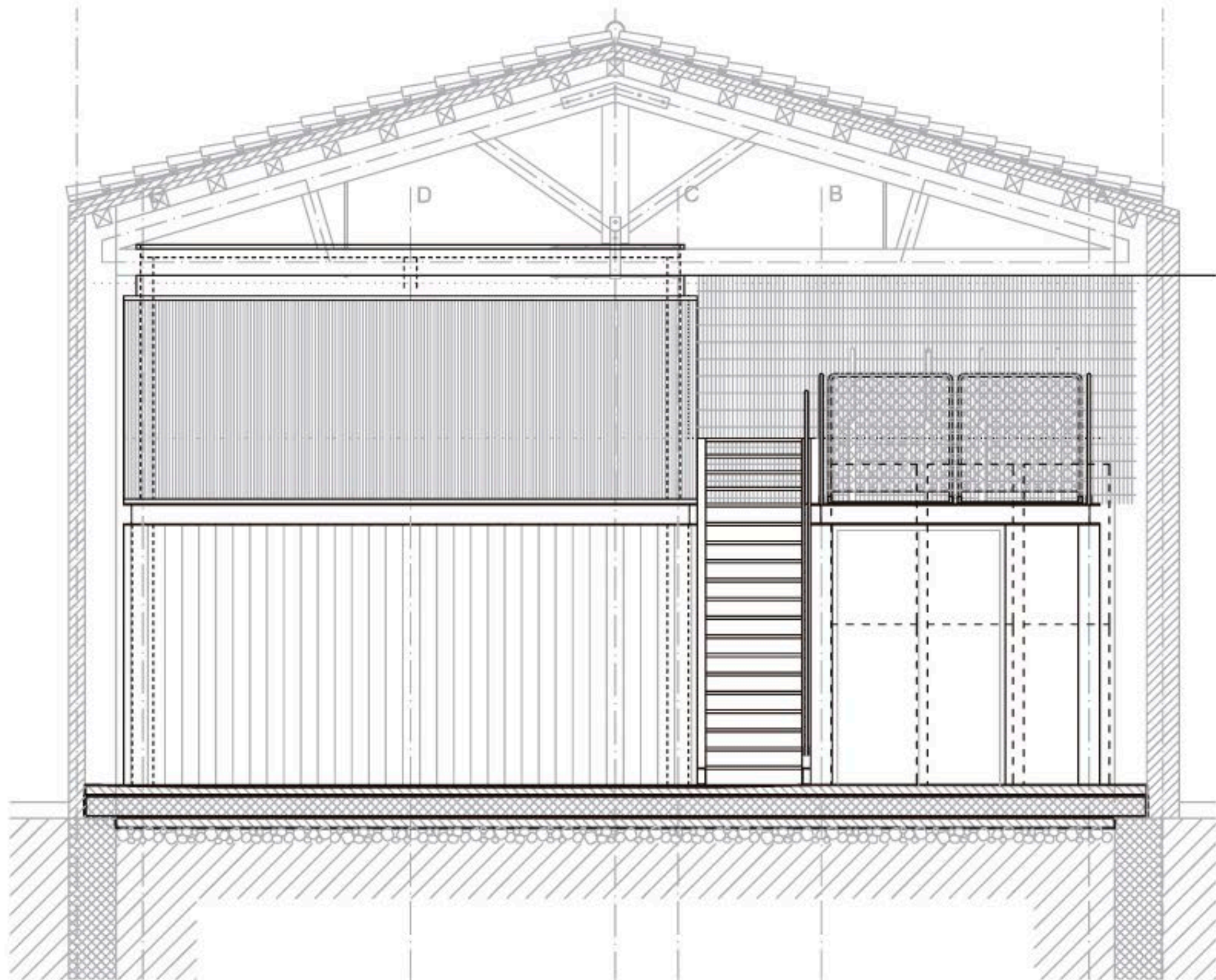
sección transversal 1
