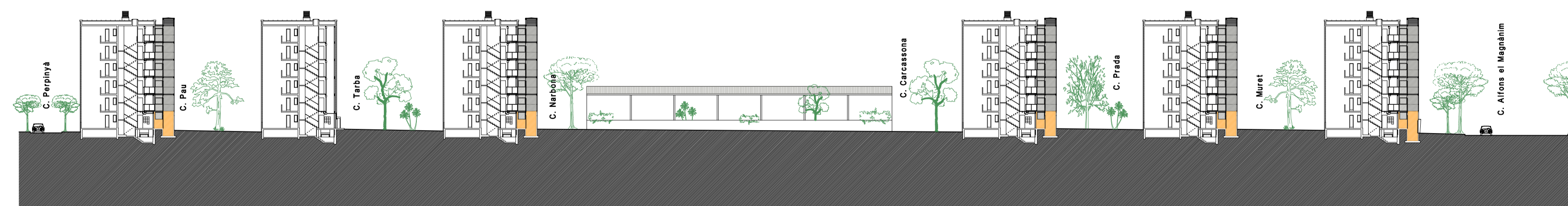
SECCION DEL SECTOR DE BLOQUES TIPO 2
