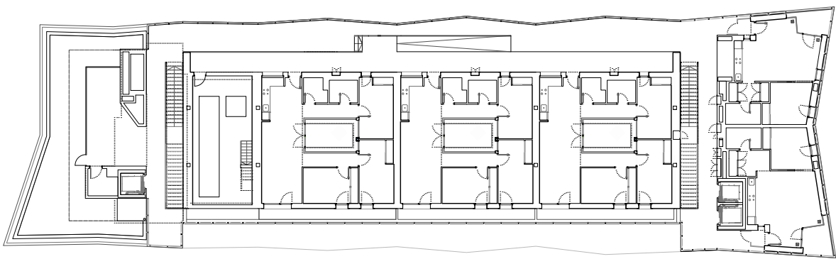
PLANTA ÁTICO
