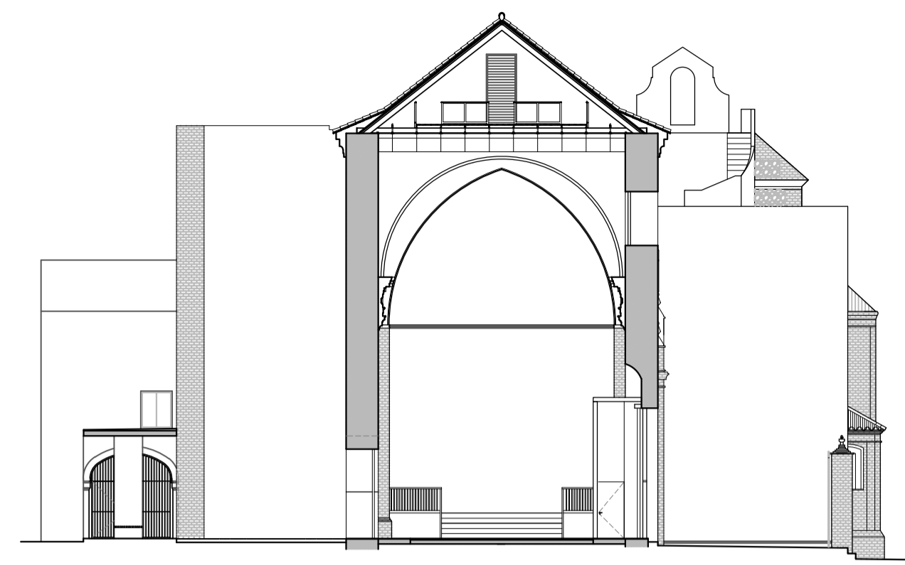
Sección 2
