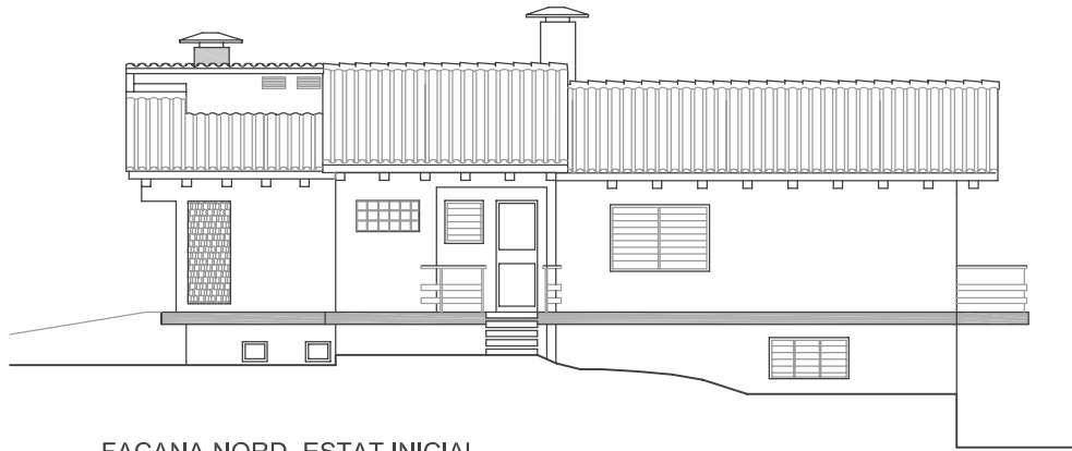
FAÇANA NORD. ESTAT INICIAL
