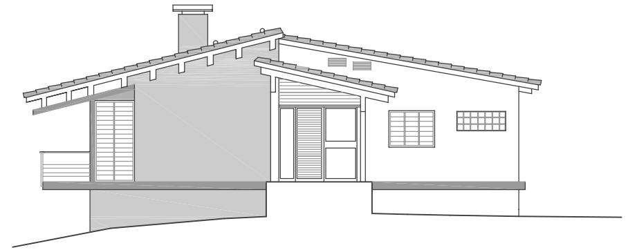
FAÇANA LLEVANT. ESTAT INICIAL
