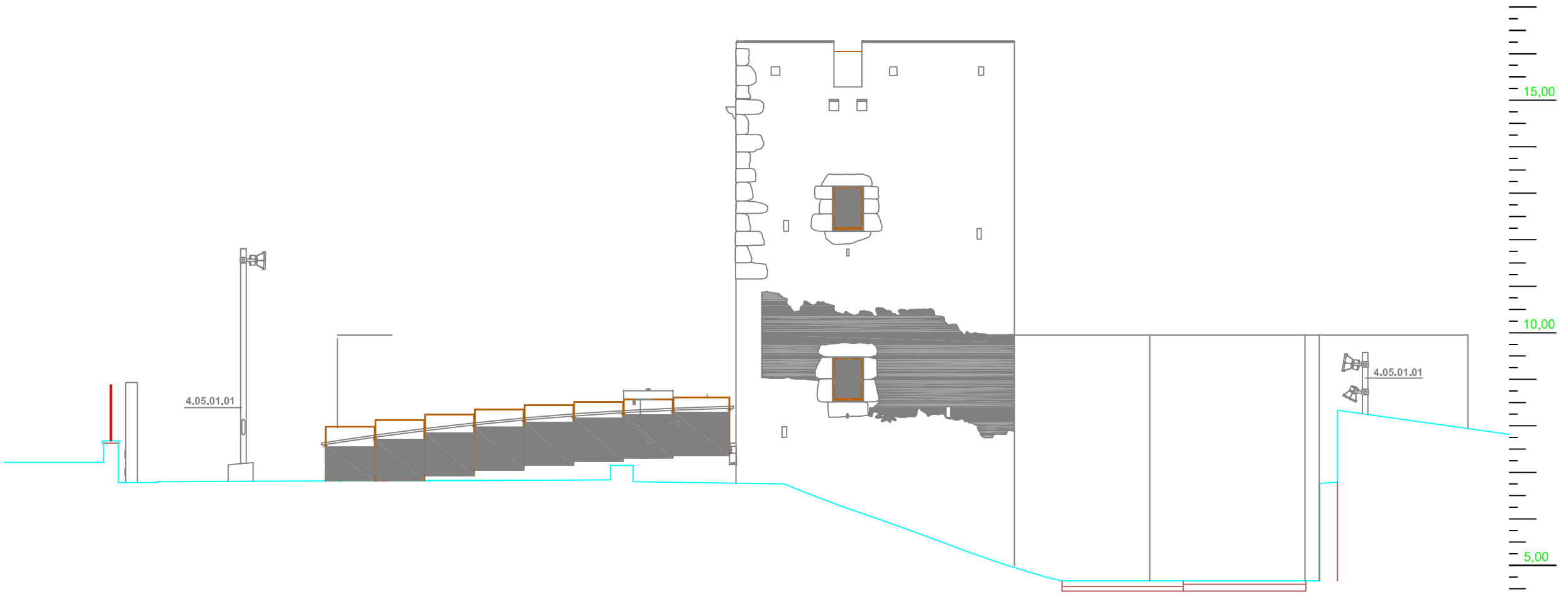
ALÇAT OEST - SECCIÓ D-D'
